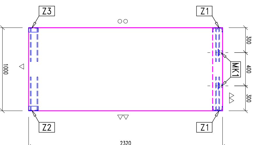
POHLED 2
